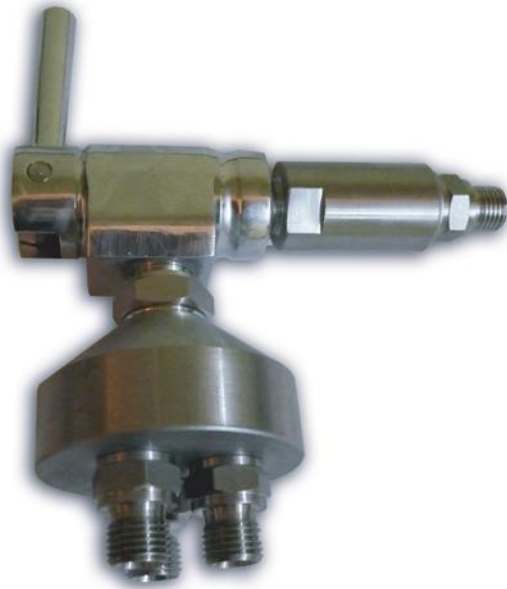
Válvula de palanca sin prefiltro 1/4" - 5/8"
